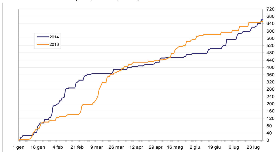
Grafico 9 – Cumulata delle precipitazioni (in mm) da inizio anno 2014 e 2013
