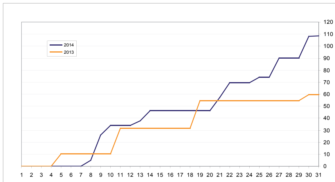
Grafico 8 – Cumulata delle precipitazioni (in mm) per luglio 2014 e 2013
