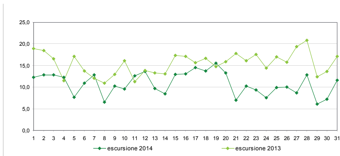
Grafico 6 – Escursione termica giornaliera (Tmax – Tmin). Mese di luglio 2014 e 2013
